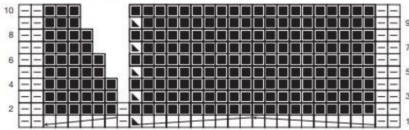
GRILLE 3 (diminutions sur la droite, taille M)
